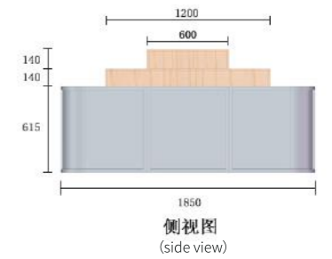
内部支架结构
