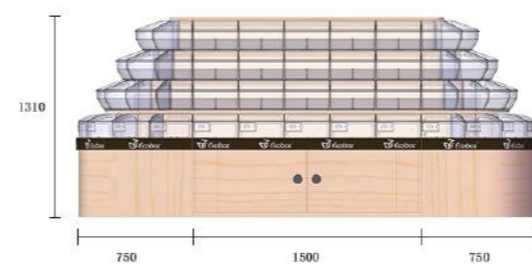
正面视图 (Front View)
