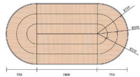
俯视图 (Top View)
