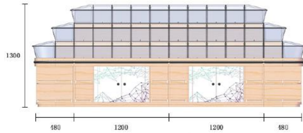
正面视图 (Front View)
