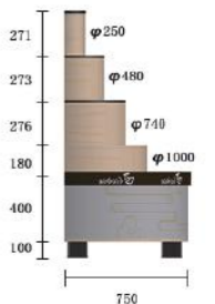
端柜侧视图 (side view)
