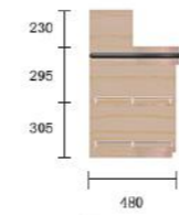
端柜侧视图 (side view)
