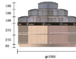
端面视图 (End View)
